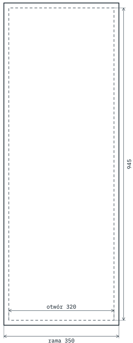
PODTYNKOWA — rama i otwór w ścianie
